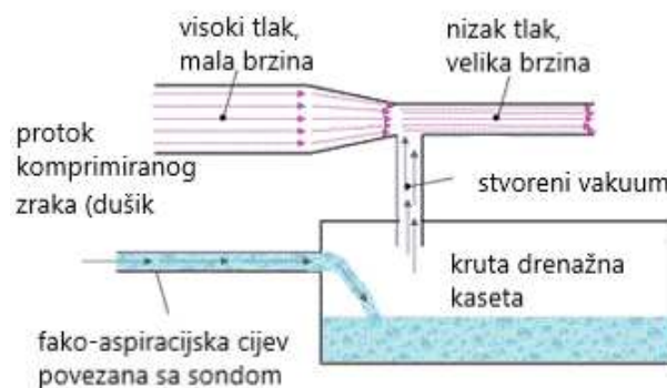
Slika 4: Venturi pumpa za fakoemulzifikaciju
