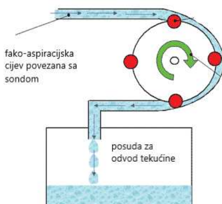
Slika 5: Peristaltička pumpa za fakoemulzifikaciju
