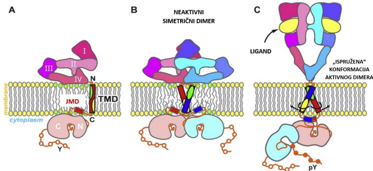
Slika 4. Mehanizam aktivacije EGF receptora. Slika A prikazuje inaktivni monomer receptora. Slika B prikazuje simetrični (neaktivni) dimer. Slika C prikazuje aktivnu konformaciju dimera EGF receptora vezanih za ligand i posljedičnu fosforilaciju tirozinskih ostataka C-terminalnog repa. Preuzeto s Bocharov EV, Lesovoy DM, Pavlov KV, Pustovalova YE, Bocharova OV, Arseniev AS. Alternative packing of EGFR transmembrane domain suggests that protein-lipid interactions underlie signal conduction across membrane. Biochim Biophys Acta-Biomembranes . 2016;1858:1254-61.
