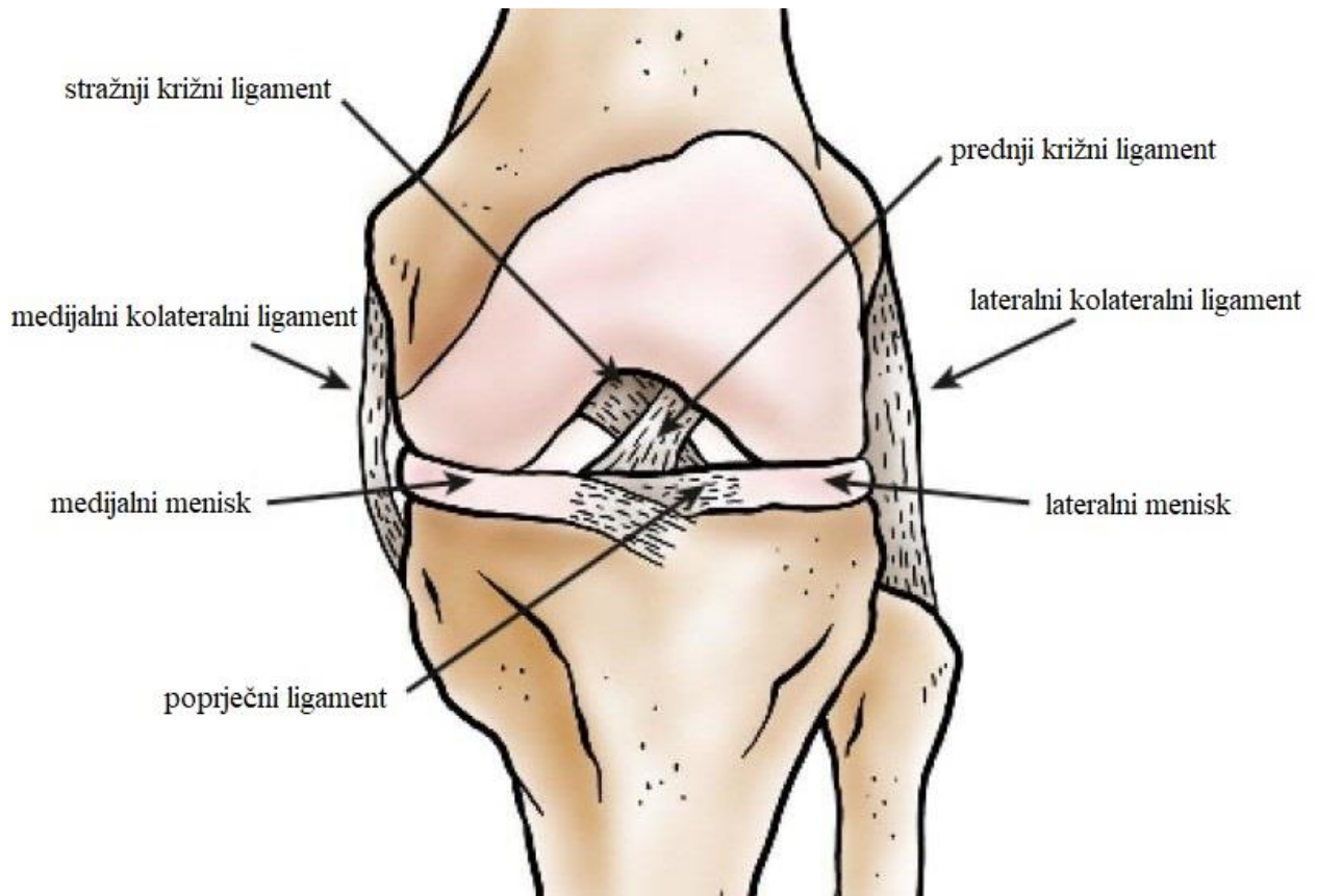
Slika 1. Menisci i zglobne sveze koljena. (Preuzeto: Makris A, Hadidi P, Athanasiou KA. Biomaterials. 2011.)
