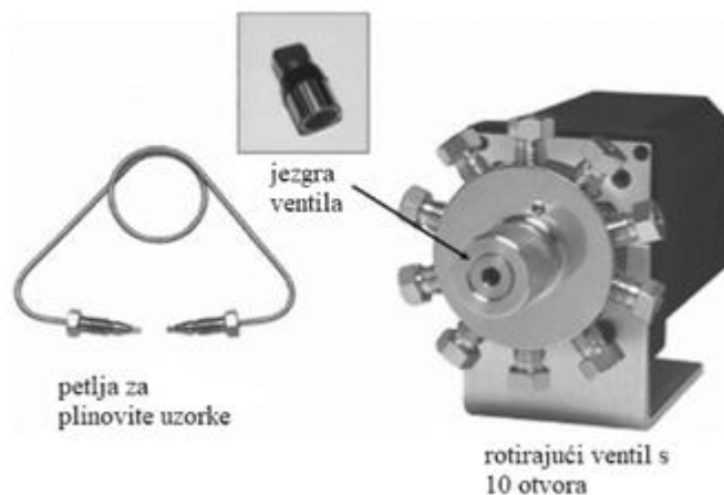
Slika 1.4. Rotirajući ventil za unošenje plinovitog uzorka s 10 otvora i petlja za plinovite uzorke. Jezgra ventila se nalazi u unutrašnjosti i rotira se kako bi promijenila smjer protoka u ventilu. Petlja za plinovite uzorke se može ugraditi na ventil, a služi za prijenos određene količine plina na kolonu (11).
