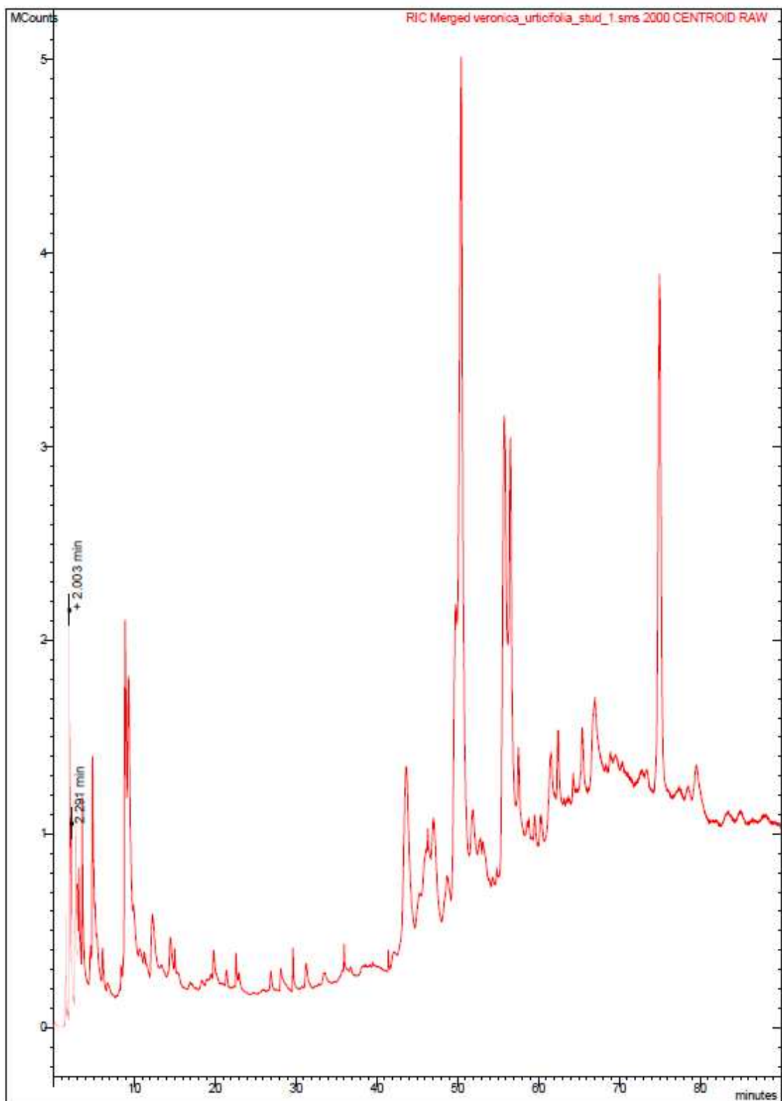
Graf 6. Kromatogram ukupne ionske struje za hidrolat vrste Veronica urticifolia Jacq. (Lokalitet 2) na koloni VF-5 MS. Najzastupljeniji spoj je heksahidrofarnezil aceton.
