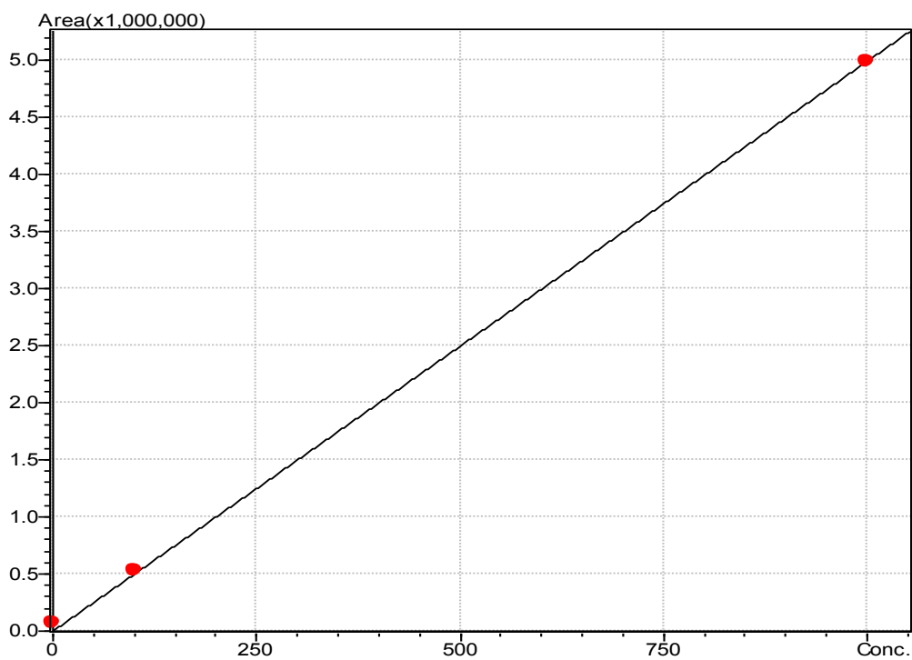
Slika 20. Baždarna krivulja za kotinin u koncentracijskom području od 0-1000 ng/mL
