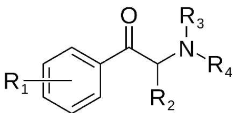
Slika 34. Opća struktura katinona
