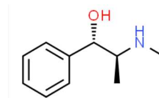
Slika 86. Pseudoefedrin
