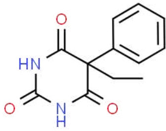
Slika 12. Fenobarbital (11)
