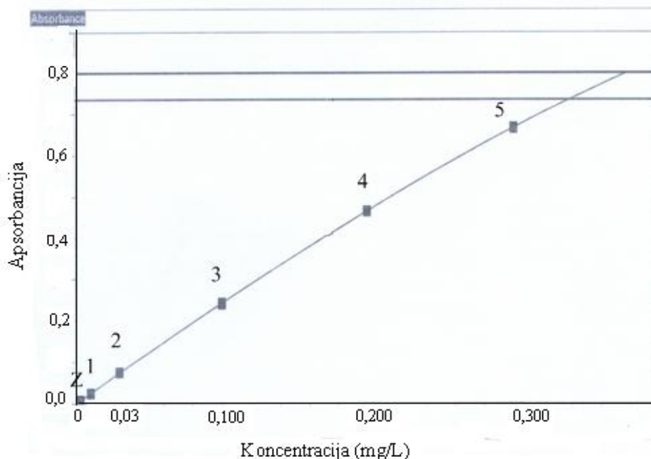
Slika 2.3. Kalibracijski pravac za živu. Apcisa predstavlja koncentraciju radnih otopina standarda žive (Hg) izraženu u \text{mg/L} : Z–0; 1–0,01; 2–0,03; 3–0,1; 4–0,2; 5–0,3. Ordinata predstavlja apsorbanciju svjetlosti (intenzitet svjetlosti prije i poslije propuštanja kroz analit).
