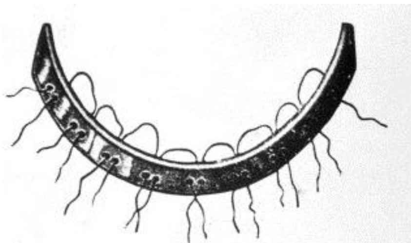
Slika 1. Fauchardov bandeau.
