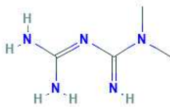
Slika 3. Struktura metformina
