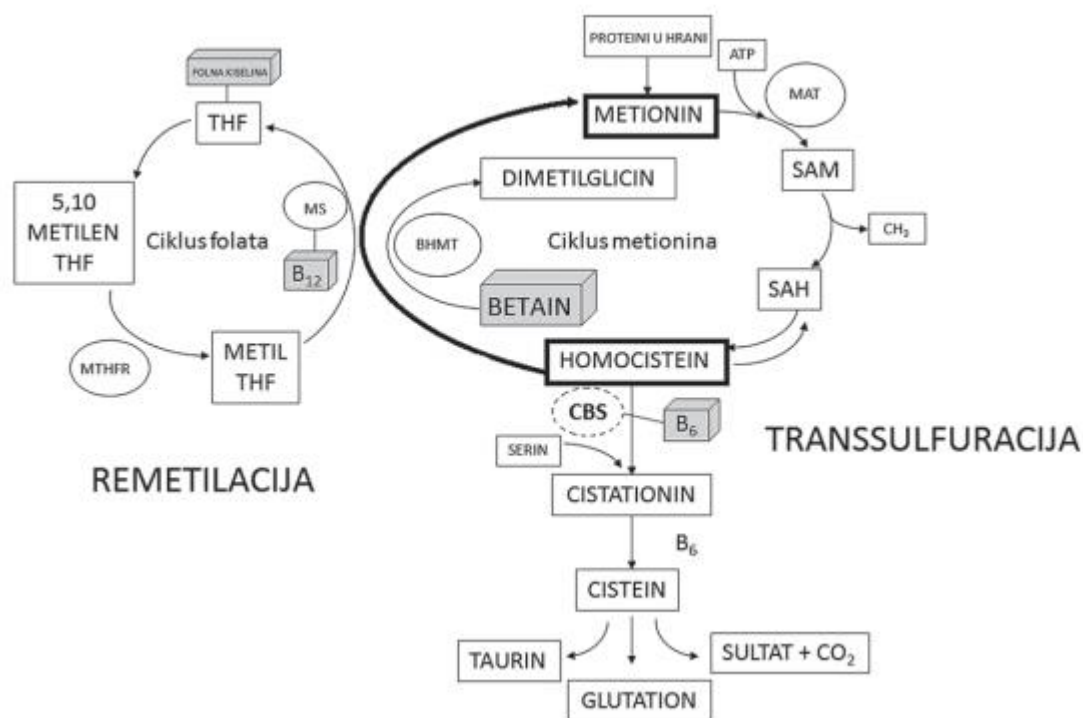
Slika 3. Sinteza metionina i glutationa. ATP-adenozin trifosfat, MAT-S-metionin adenozil transferaza, SAH-S-adenozil homocistein, CBS-cistation β-sintaza, BHMT-betain-homocistein metiltransferaza, MS-metionin sintaza, THF-5,10 metilentetrahidrofolat, MTHFR-5,10 metilentetrahidrofolat reduktaza (45).
