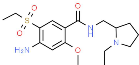
Slika 77. Amisulprid (11)
