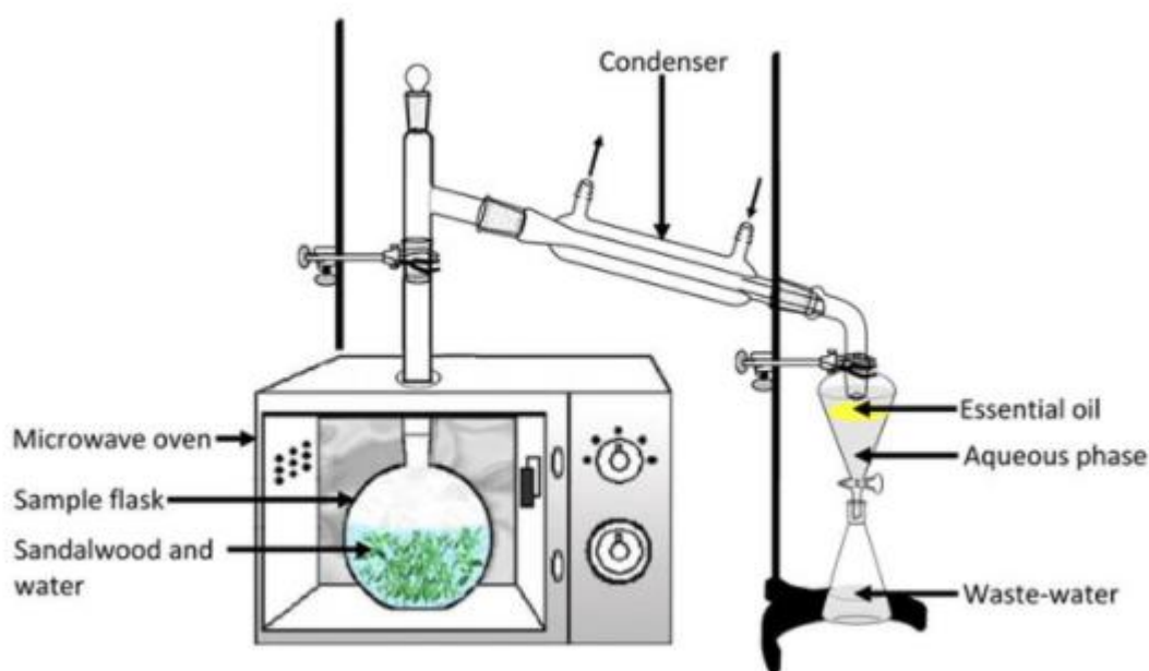
Slika 6. Uređaj za mikrovalnu ekstrakciju
