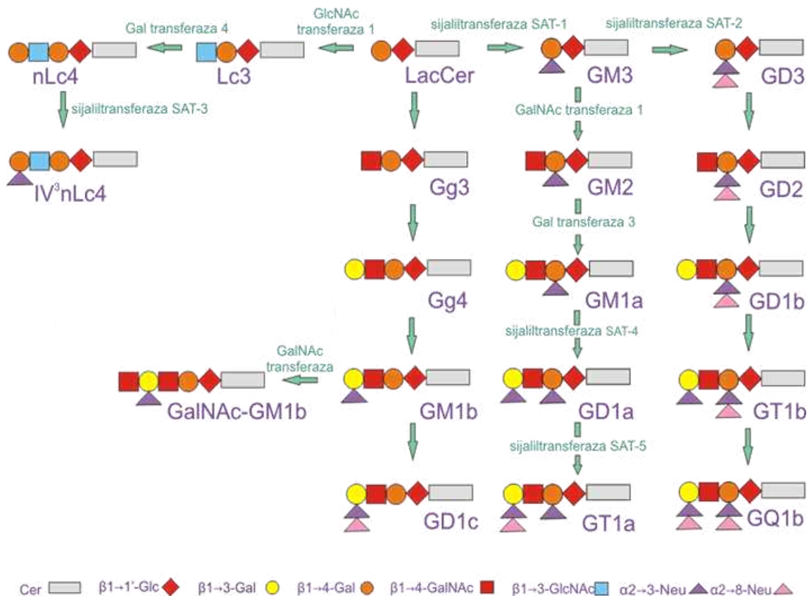
Slika 13. Osnovni putevi biosinteze ganglioserijske i neolaktoserijske gangliozida. Preuzeto iz doktorske dizertacije Čikeš Čulić (106).
