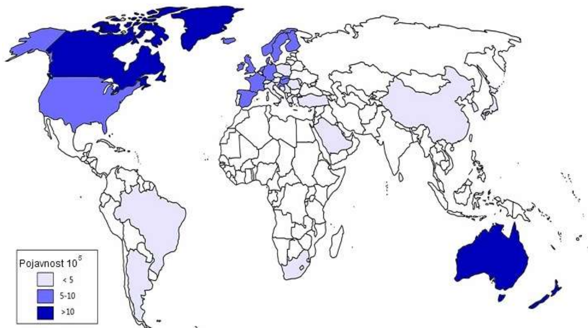
Slika 8. Globalna mapa pojavnosti Crohnove bolesti.
