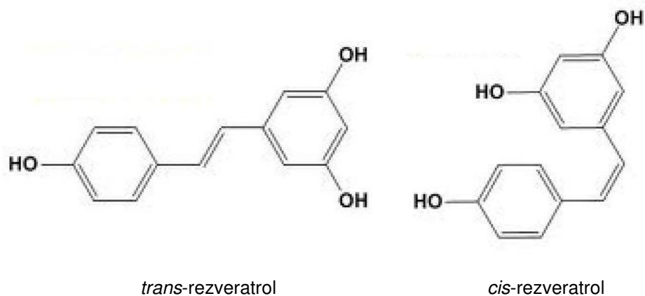
Slika 3. Izomeri rezveratrola
