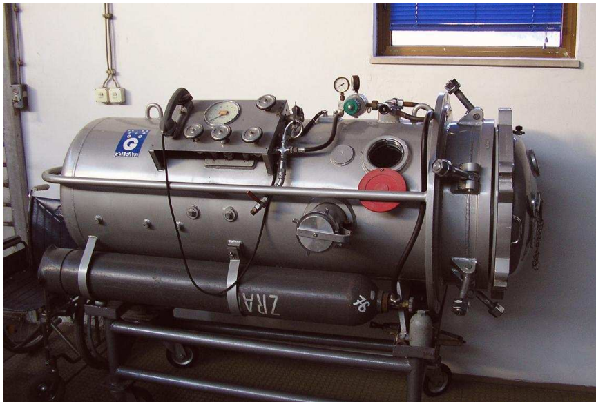
Slika 7. Jednodijelna rekompresijska barokomora
