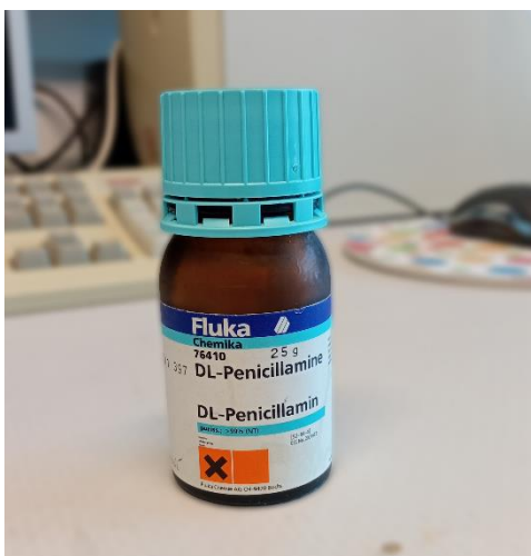
Slika 12. PEN, kemijski spoj korišten za pripravu standardne otopine.
