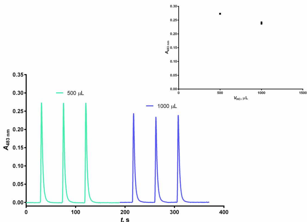
Slika 28. Siagram optimizacije volumena petlje zadržavanja. Volumen petlje zadržavanja ( V_{\text{HC}} ): a) 500 \mu\text{L} ; b) 1000 \mu\text{L} . Eksperimentalni uvjeti: c(\text{PEN}) = 4,0 \times 10^{-5} \text{ M} ; c(\text{Cu}^{2+}) = 3,2 \times 10^{-4} \text{ M} ; c(\text{BCS}) = 6,4 \times 10^{-4} \text{ M} ; \text{pH} = 5 ; Q_{\text{CS}} = 5000 \mu\text{L}/\text{min} ; V_{\text{RS}} = 150 \mu\text{L} ; V_a = 200 \mu\text{L} ; volumen protočne kivete = 30 \mu\text{L} ; l = 70 \text{ cm} ; \lambda = 483 \text{ nm} ; t = 25 \text{ }^\circ\text{C} . Umetak: ovisnost apsorbancije o volumenu petlje zadržavanja za određivanje PEN-a.
