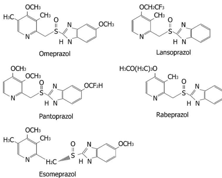
Slika 2. Kemijske strukture inhibitora protonske pumpe (22)
