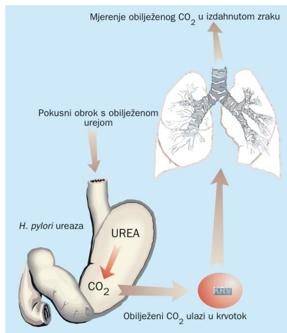
Slika 4. Princip rada ^{13}\text{C} UBT testa (36)
