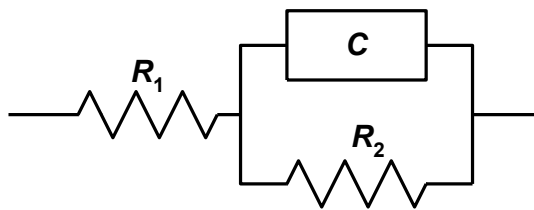
Slika 3.7. Električni ekvivalentni krug jednostavne elektrokemijske ćelije.
