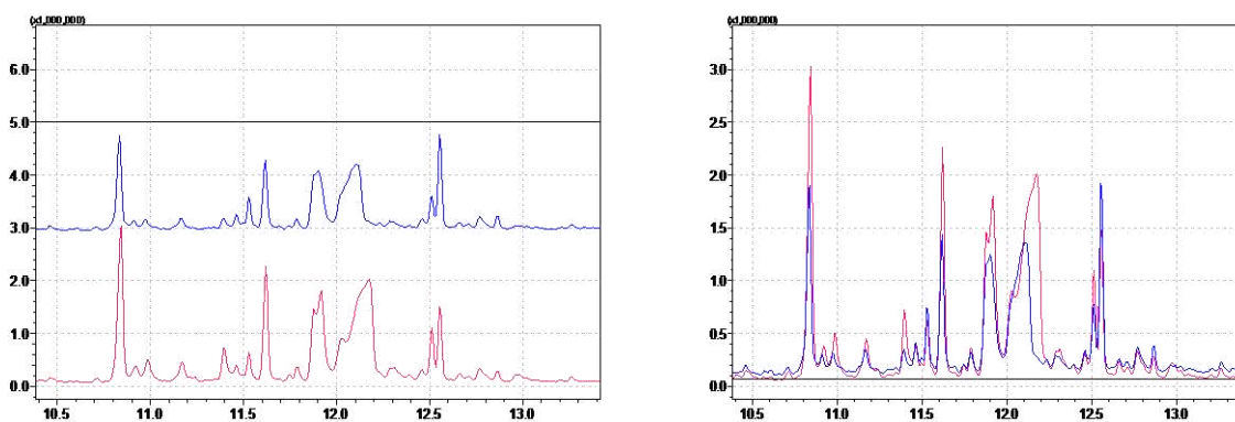
Slika 12. Usporedba signala biološkog uzorka ispitanika br. 1. Crna linija – biološki uzorak natašte, plava linija – biološki uzorak nakon 1 sata, roza linija – biološki uzorak nakon 2 sata od konzumacije Dorina čokolade za kuhanje.
