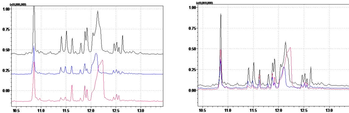
Slika 13. Usporedba signala biološkog uzorka ispitanika br. 2. Crna linija – biološki uzorak natašte, plava linija – biološki uzorak nakon 1 sata, roza linija – biološki uzorak nakon 2 sata od konzumacije Dorina čokolade za kuhanje.
