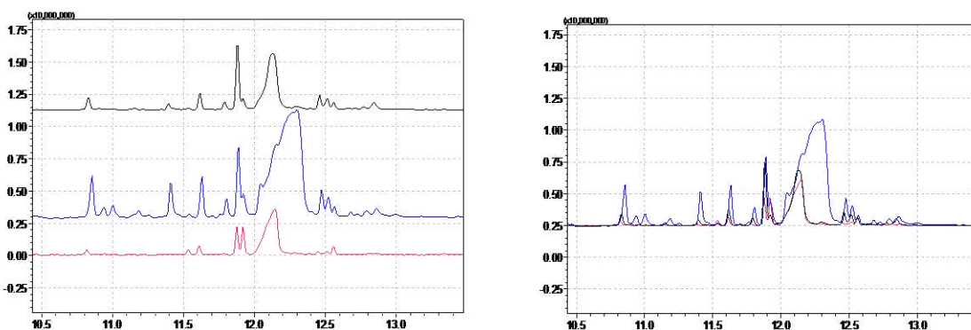
Slika 14. Usporedba signala biološkog uzorka ispitanika br. 3. Crna linija – biološki uzorak natašte, plava linija – biološki uzorak nakon 1 sata, roza linija – biološki uzorak nakon 2 sata od konzumacije Dorina čokolade za kuhanje.
