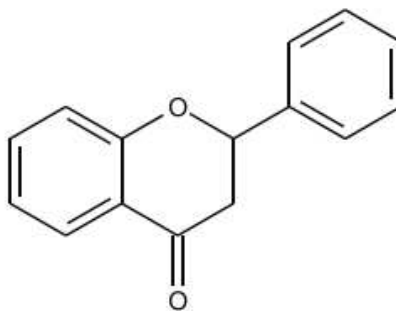
Slika 4. Struktura flavanona (8).
