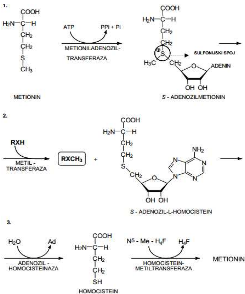
Slika 16. Mehanizam reakcije metilacije (9).
