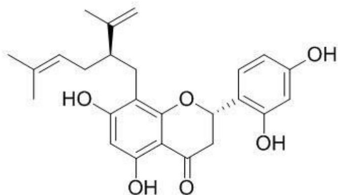
Slika 31. Struktura soforaflavanona (41).
