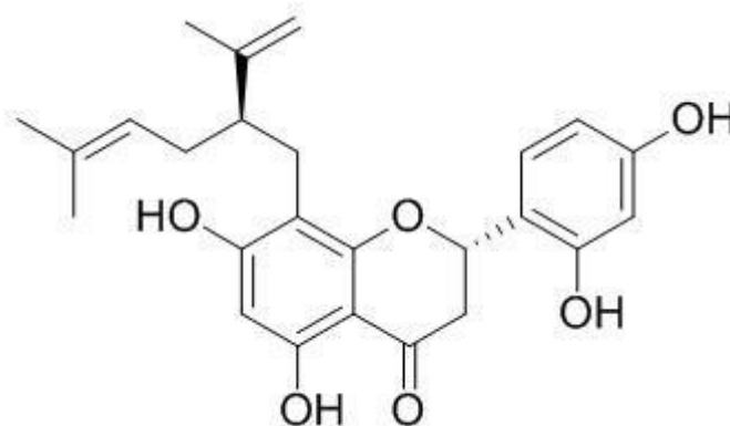
Slika 31. Struktura soforaflavanona (41).
