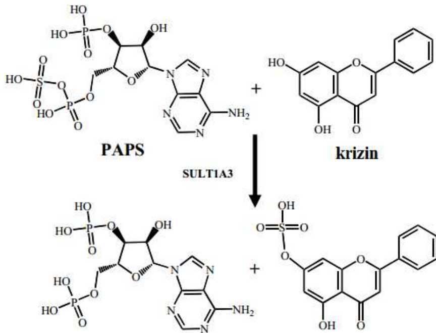
Slika 29. Sulfokonjugacija krizina (10).
