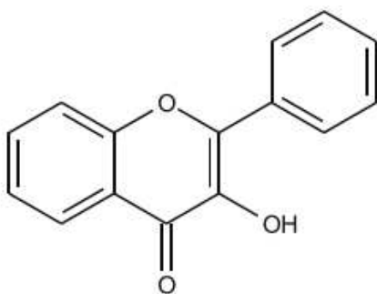
Slika 6. Struktura flavonola (8).
