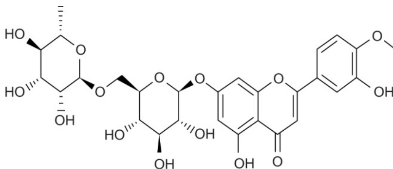
Slika 34. Struktura diosmina (68).
