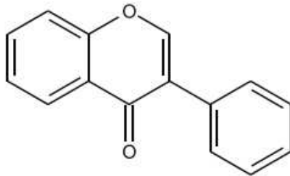
Slika 7. Struktura izoflavona (8).
