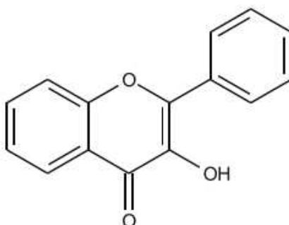
Slika 6. Struktura flavonola (8).
