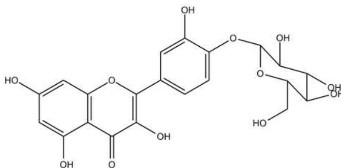
Slika 17. Struktura kvercetin-4'-O-glukozida (19).
