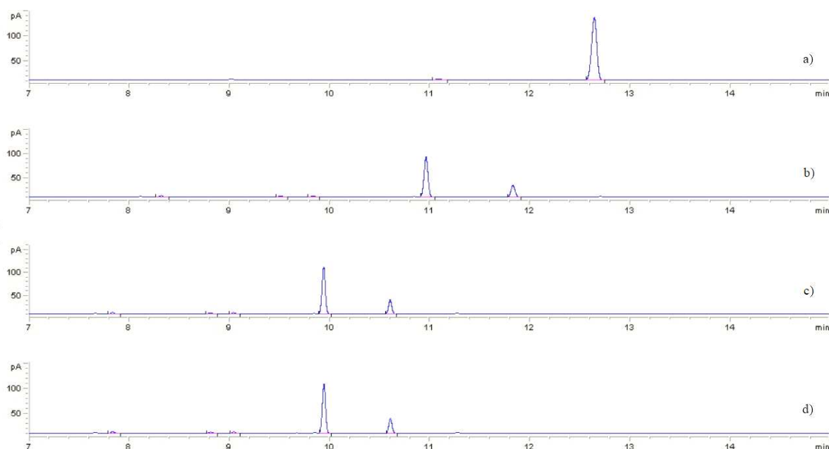
Slika 5.2. Prikaz usporedbe vremena zadržavanja limonena mjerenog različitim metodama na primjeru dobivenih kromatograma eteričnog ulja mandarine: a) metoda 1; b) metoda 2; c) metoda 3; d) metoda 4
