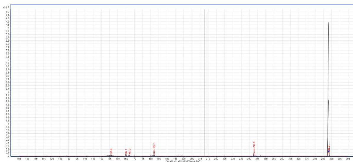
Slika 4.3. Maseni spektar zolmitriptana pri energiji sraza 20 eV
