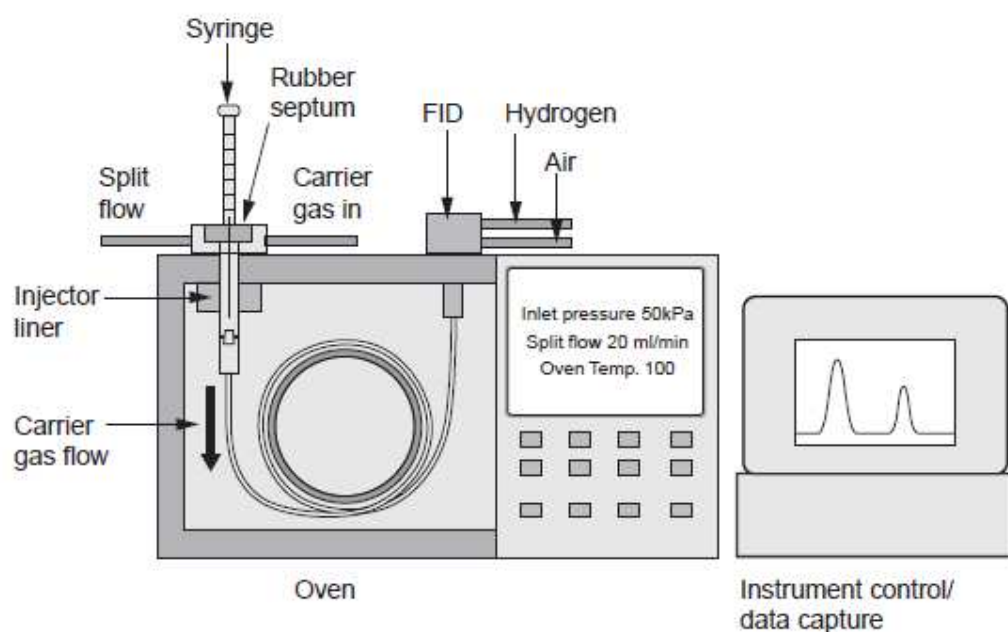
Slika 8. Shematski prikaz plinskog kromatograma (67)
