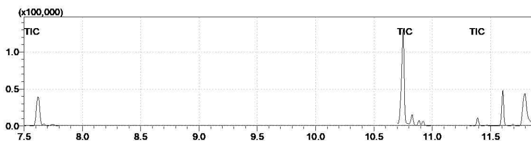
Slika 17. Prikaz dijela ukupni ionski kromatogram nikotina, kotinina, 3OHK, za uzorak 46 analiziran GC-MS metodom, s karakterističnim signalima i retencijskim vremenima izraženim u minutama; nikotin (RT =7,619), kotinin (RT=10.752) i 3-OHK (RT=11,390).
