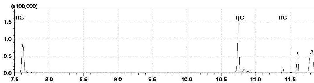
Slika 19. Prikaz dijela ukupni ionski kromatogram nikotina, kotinina, 3OHK, za uzorak 48 analiziran GC-MS metodom, s karakterističnim signalima i retencijskim vremenima izraženim u minutama; nikotin (RT =7,619), kotinin (RT=10.753) i 3-OHK (RT=11,391)
