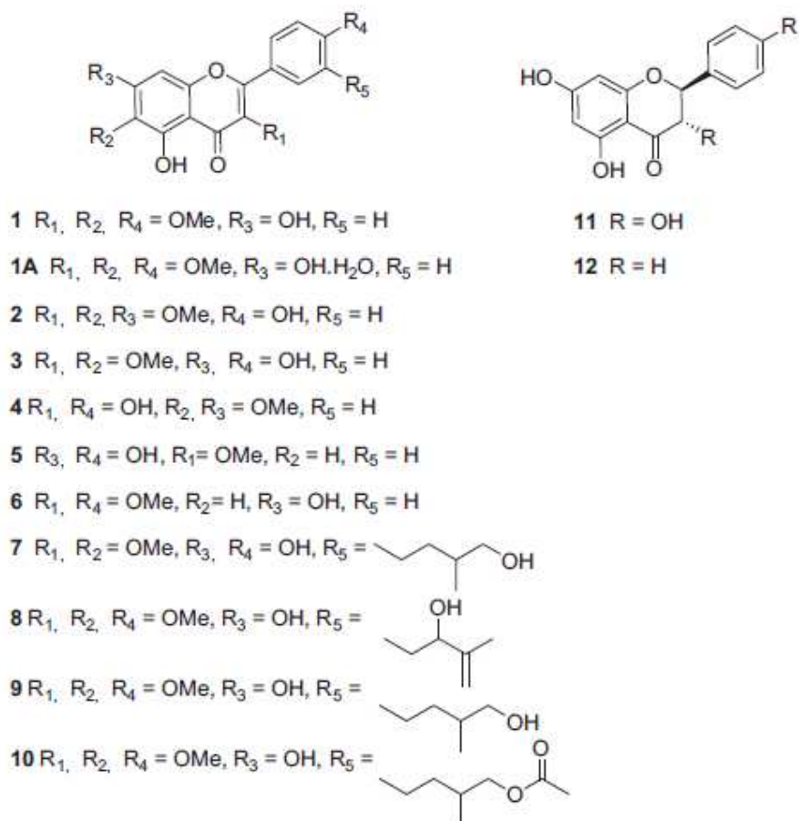
Slika 17. Strukture izoliranih flavonoida iz biljke Dodonea viscosa L. (29)
